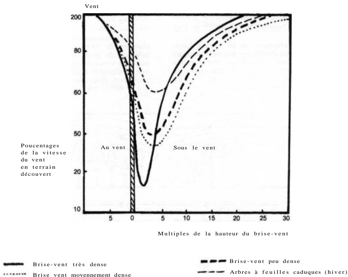
Figure 6.3.3.4 Effet d'un brise-vent protecteur en fonction de sa pénétrabilité (d'après Geiger, 31).
