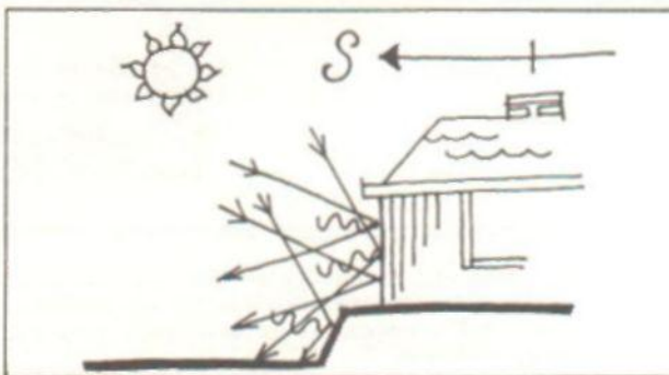
Figure 6.3.6.1 Eléments utiles pour l'accroissement du rayonnement et l'élévation de la température Les flèches indiquent l'incidence et le réfléchissement du soleil, les lignes sinusoïdales la chaleur irradiée.
