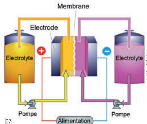
07 Principe de fonctionnement d'une batterie à redox flow . Les électrodes sont formées de liquides en mouvement, les électrolytes, séparés par une membrane perméable aux ions.
